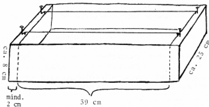
Abb. 1: Selbstbau-Monochord
