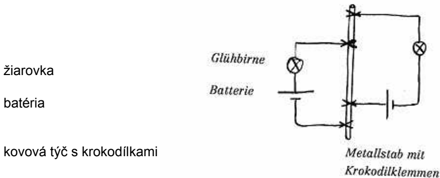
Abb. 50: Unabhängige Stromkreise überschneiden sich am selben Metallstück
