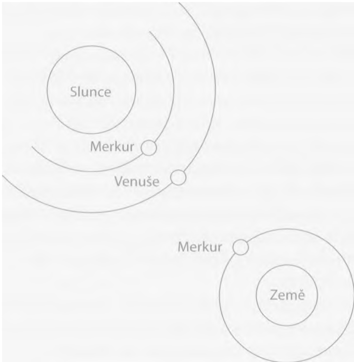
Obr. 5: Další vývoj sluneční soustavy
